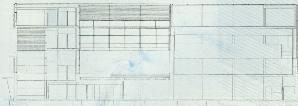
Sección HH.
