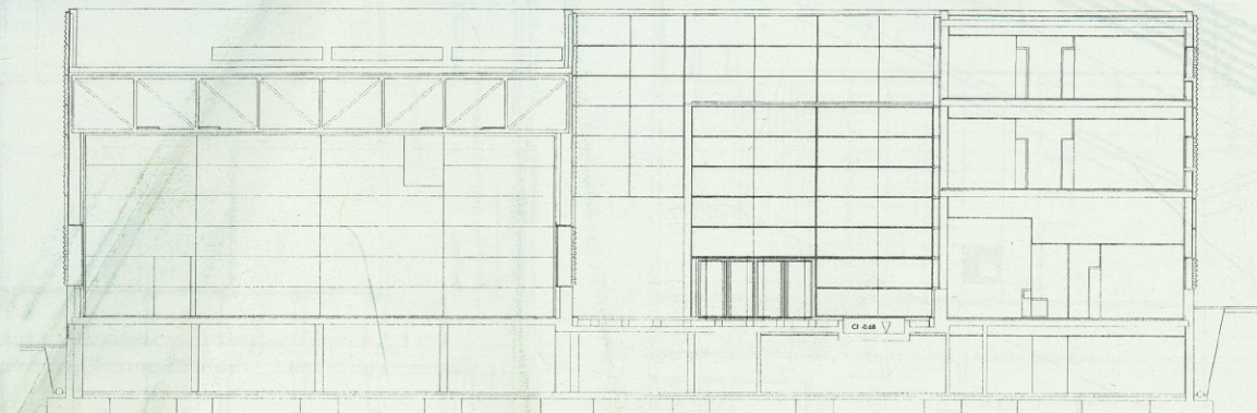
Sección GG.
