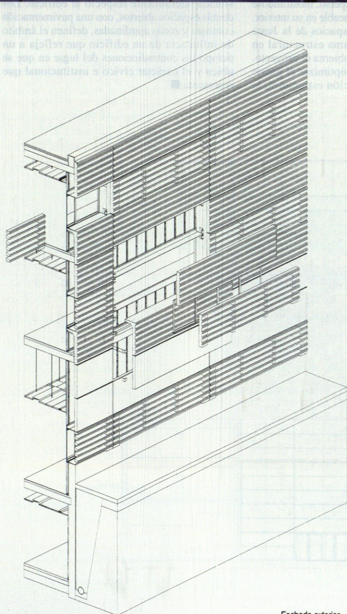
Fachada exterior.
