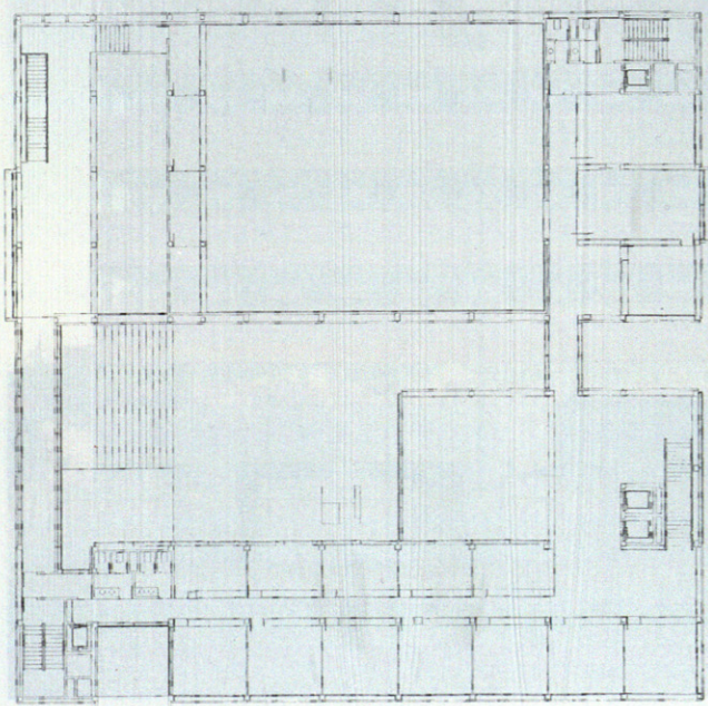
Planta primera.
